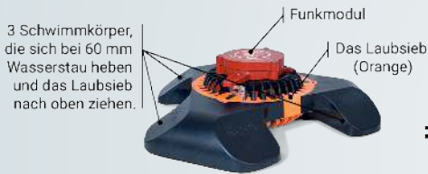
Der ROOFGUARD: Ein patentiertes Laubsieb mit Lift-Funktion und Funkmodul.
