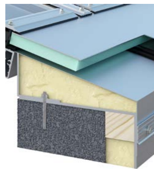
Montage auf Betonaufkantung
