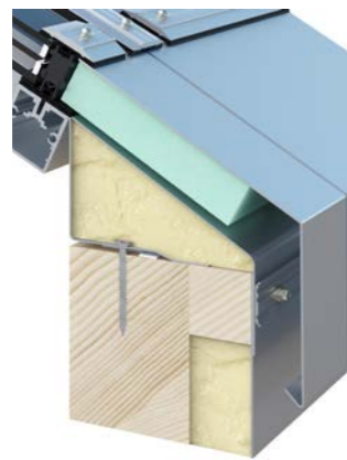
Montage auf Holzaufkantung
